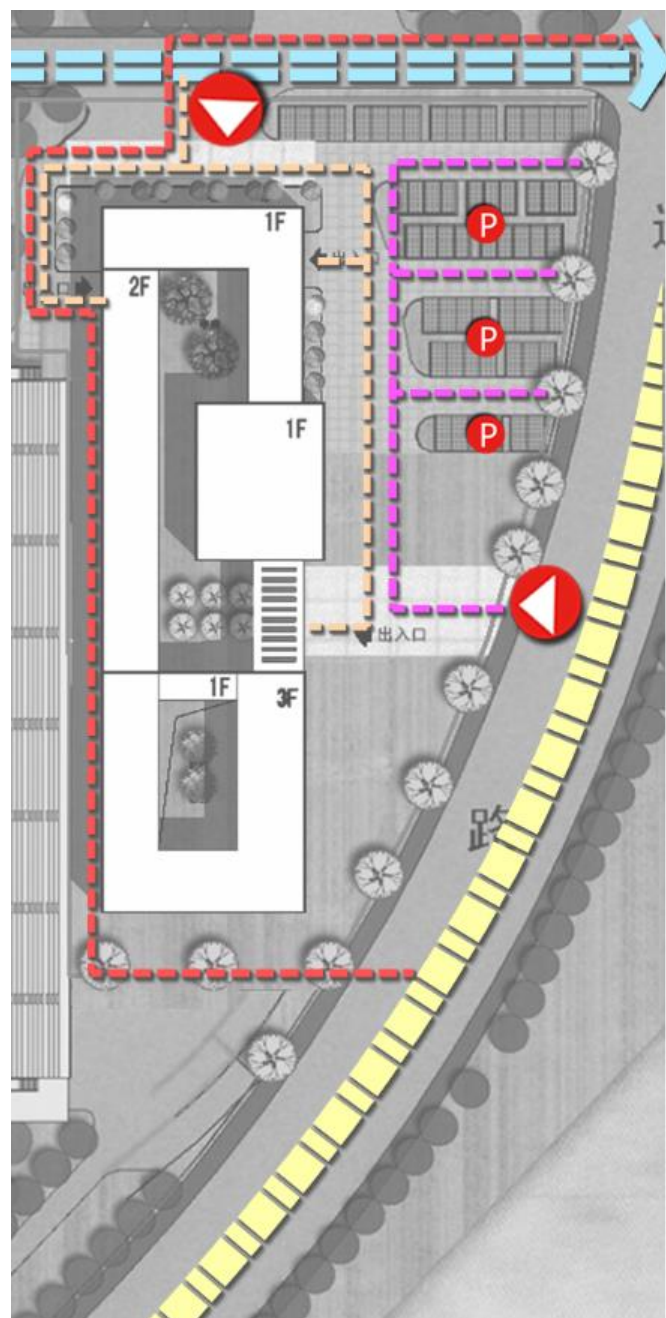
附图 5 建设项目平面布置
